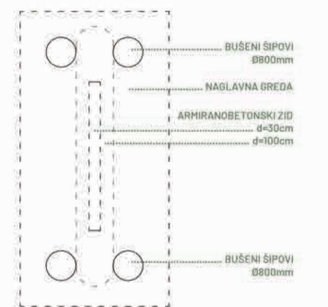
DETALJ TEMELJA 1:100
