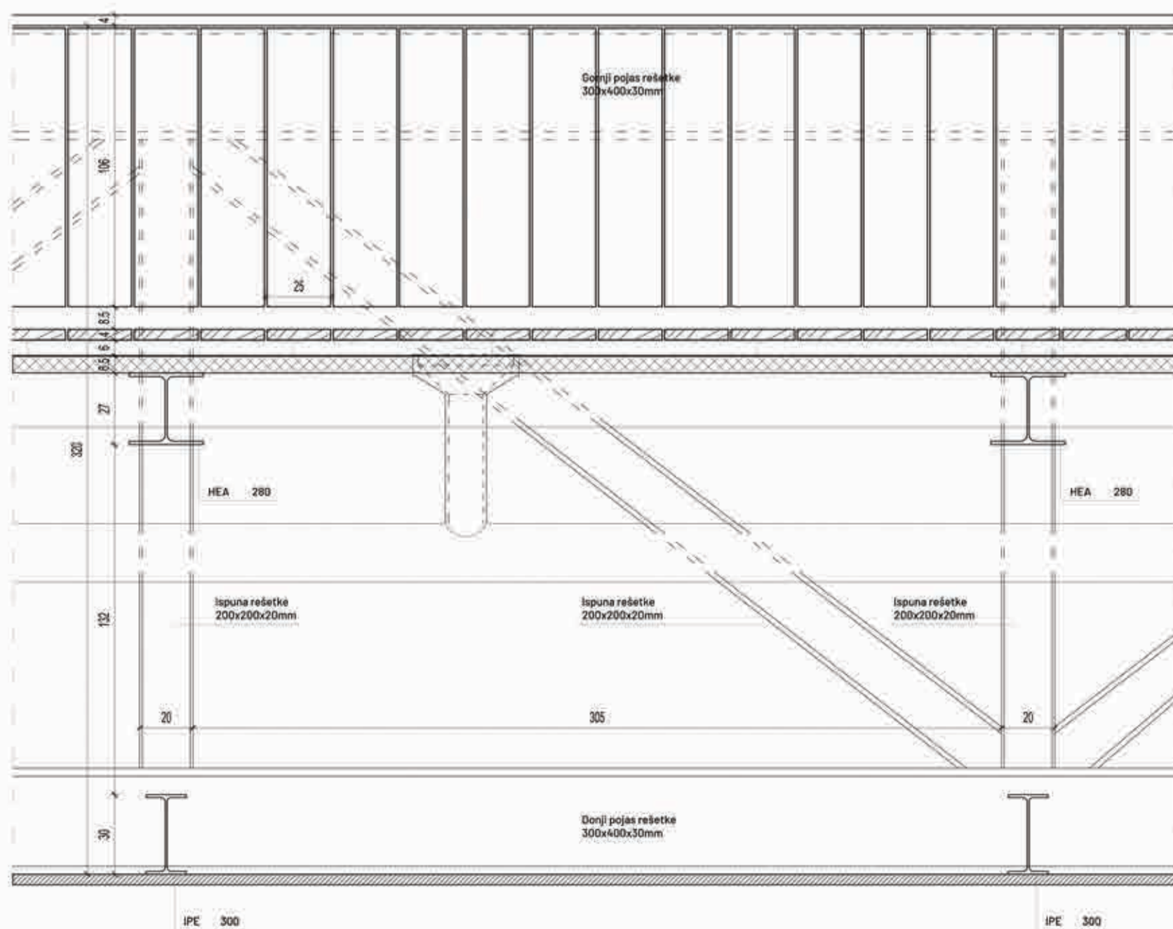
PODUŽNI PRESEK 1:20
