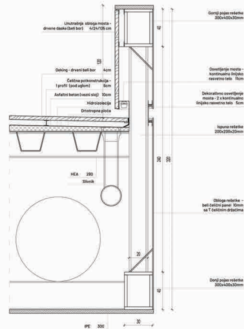
POPREČNI PRESEK KROZ OGRADU 1:20
