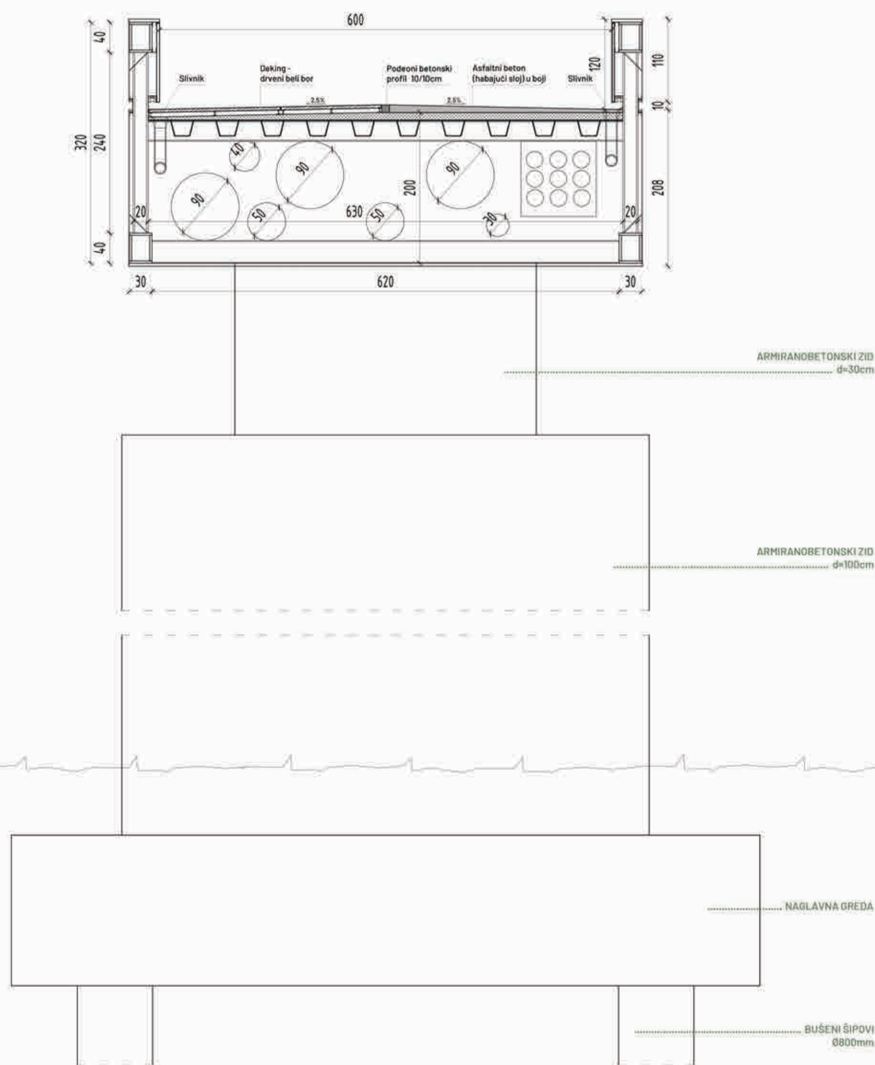
M5 - POPREČNI PRESEK MOSTA KOD STUBA U VODI 1:50
