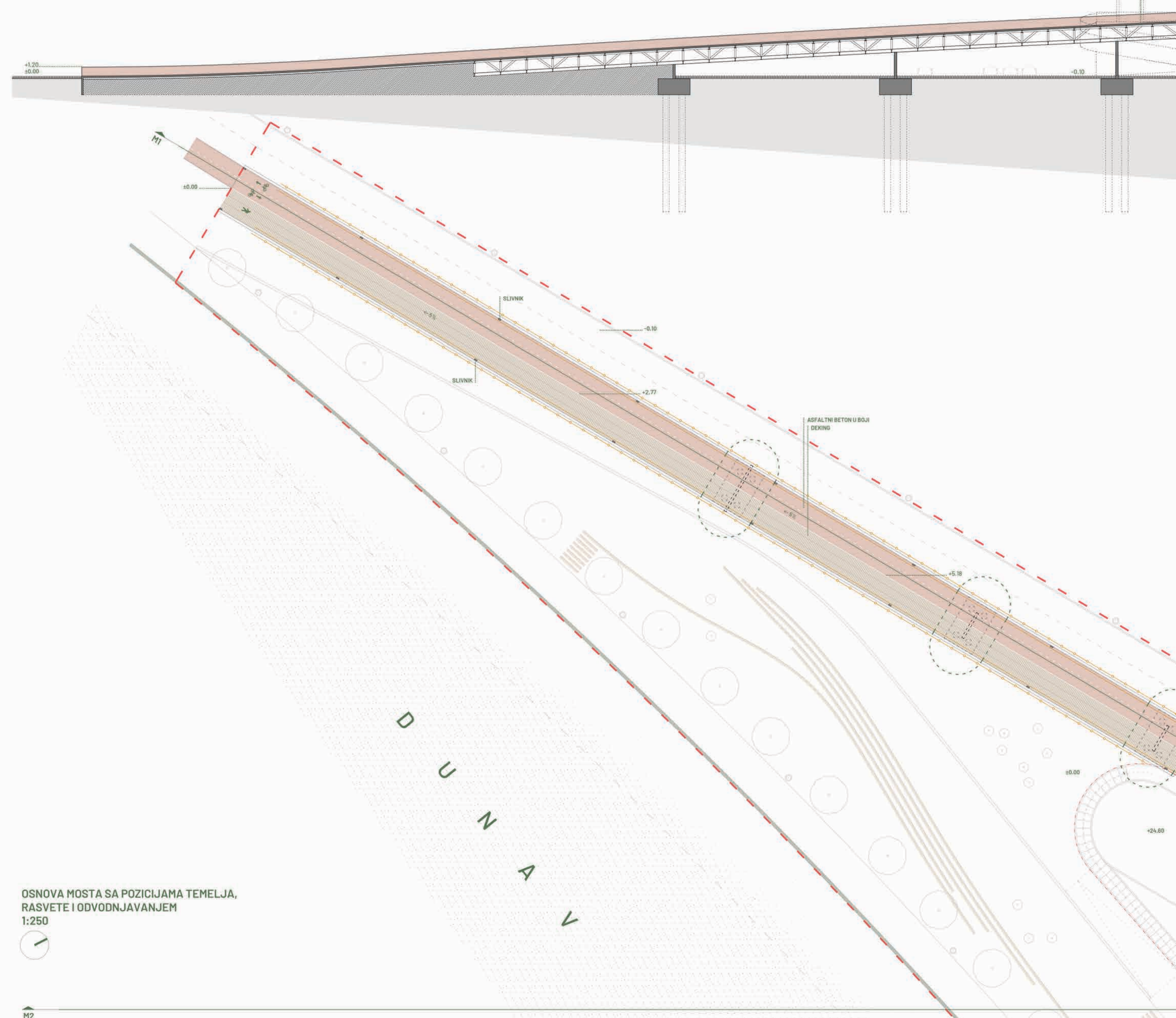
M1 - PODOŽNI PRESEK MOSTA 1:250
