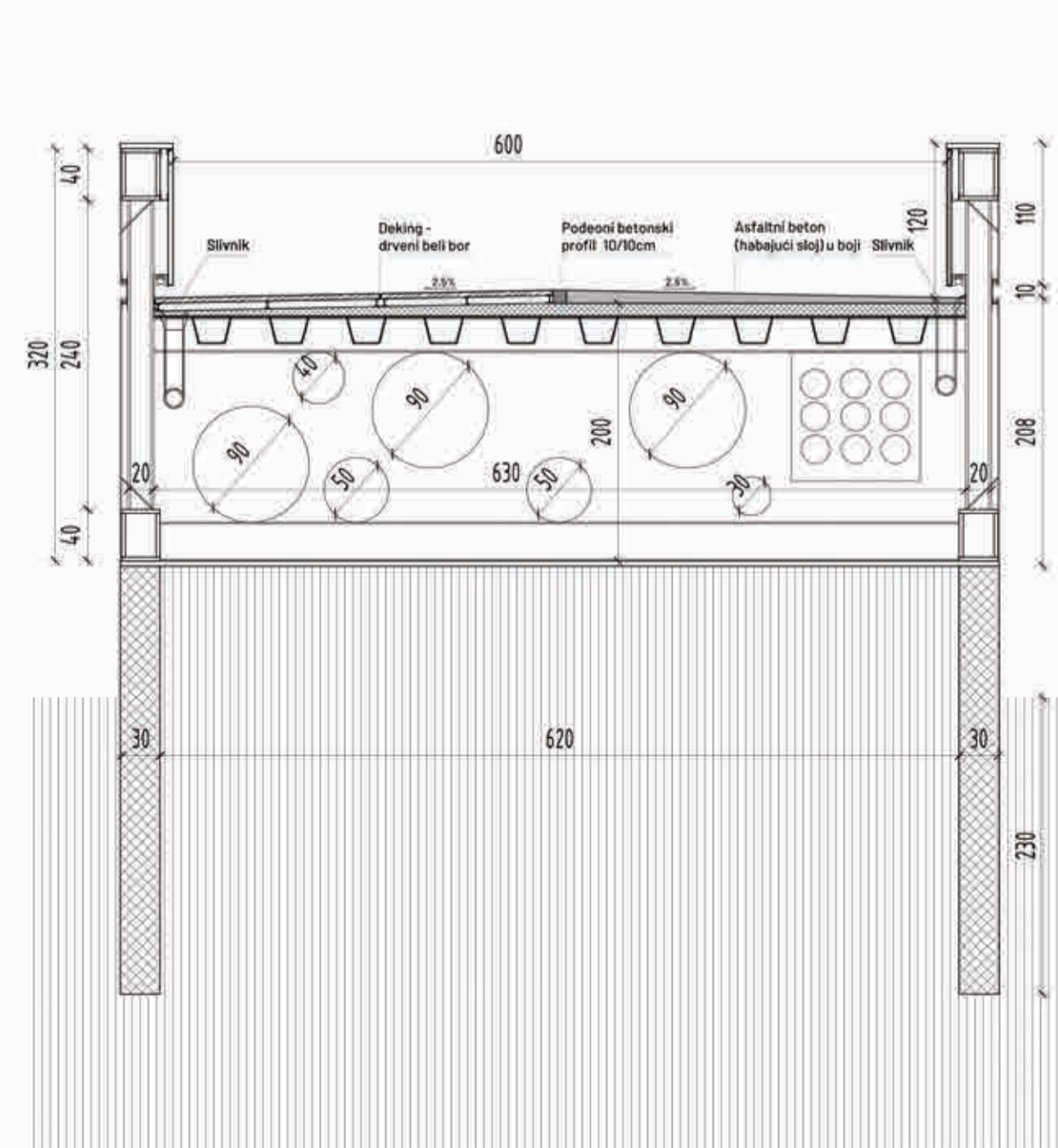
M2 - POPREČNI PRESEK KROZ NASIP 1:50
