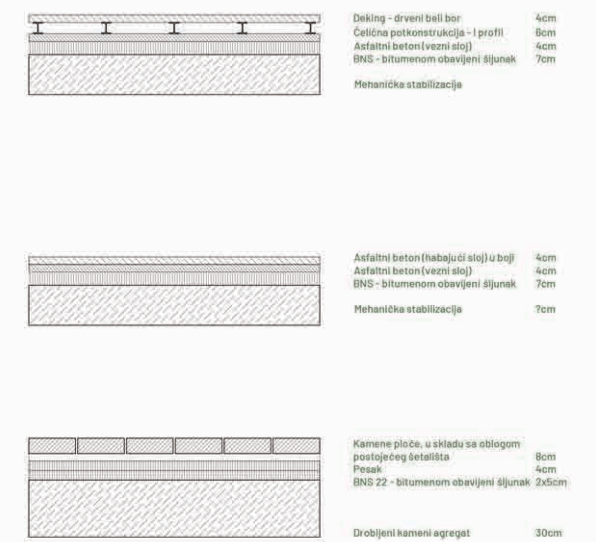
DETALJI MATERIJALIZACIJE PARTERA 1:20
